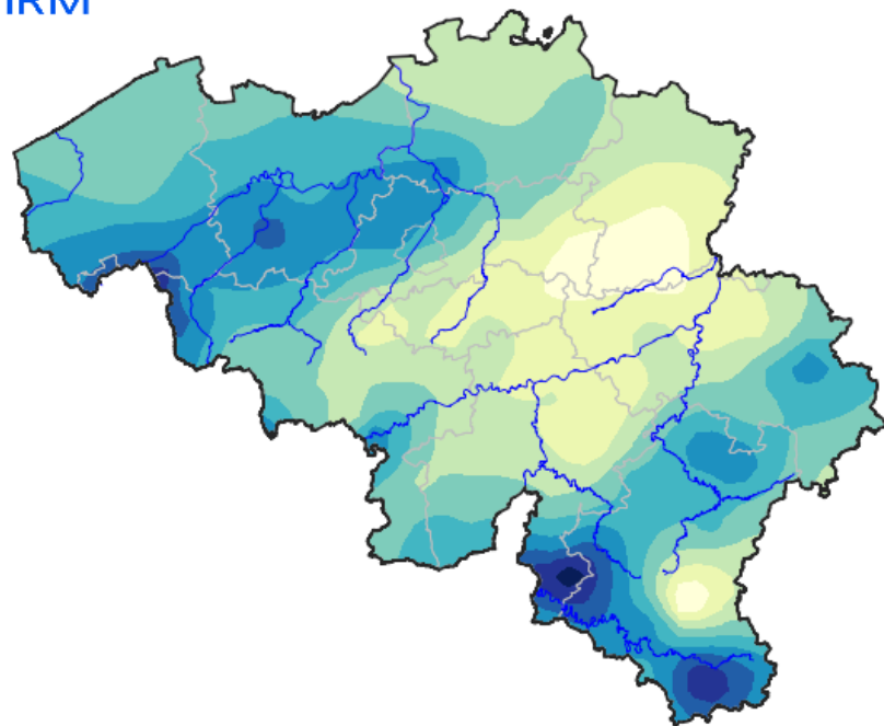
Quantités des précipitations cumul avril 2020
