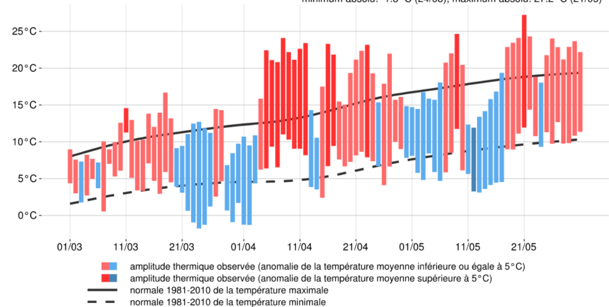
Amplitude thermique journalière, Uccle, printemps 2020
