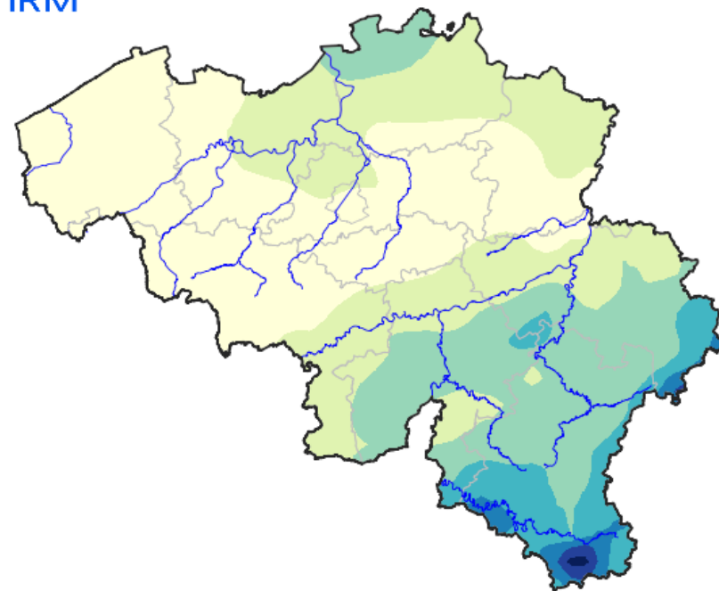
Quantités des précipitations cumul mai 2020
